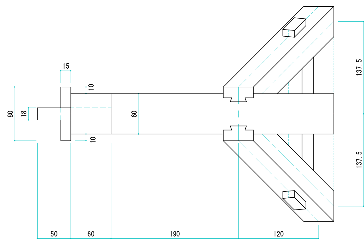
平面図
