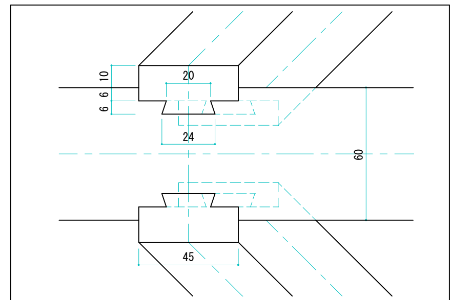
柱脚・頭繋ぎ取り付け部詳細図
