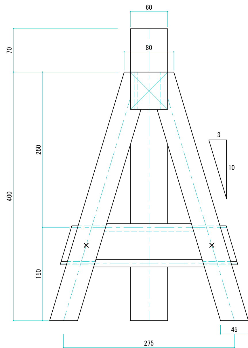
正面図
