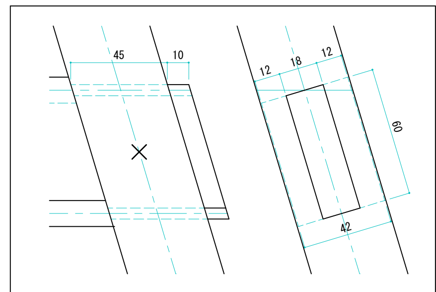
貫・柱脚取り付け部詳細図
