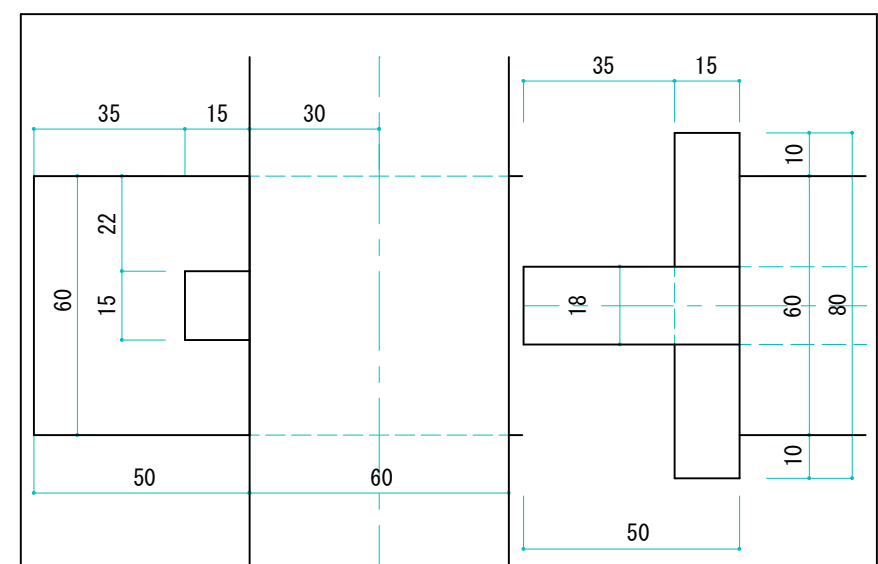
束柱・頭繋ぎ取り付け部詳細図
