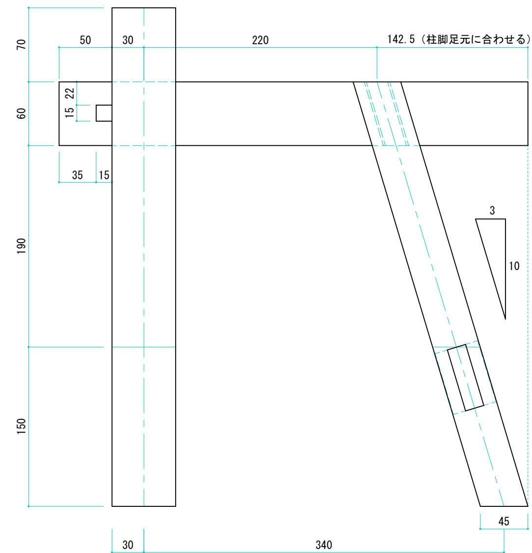
側面図
